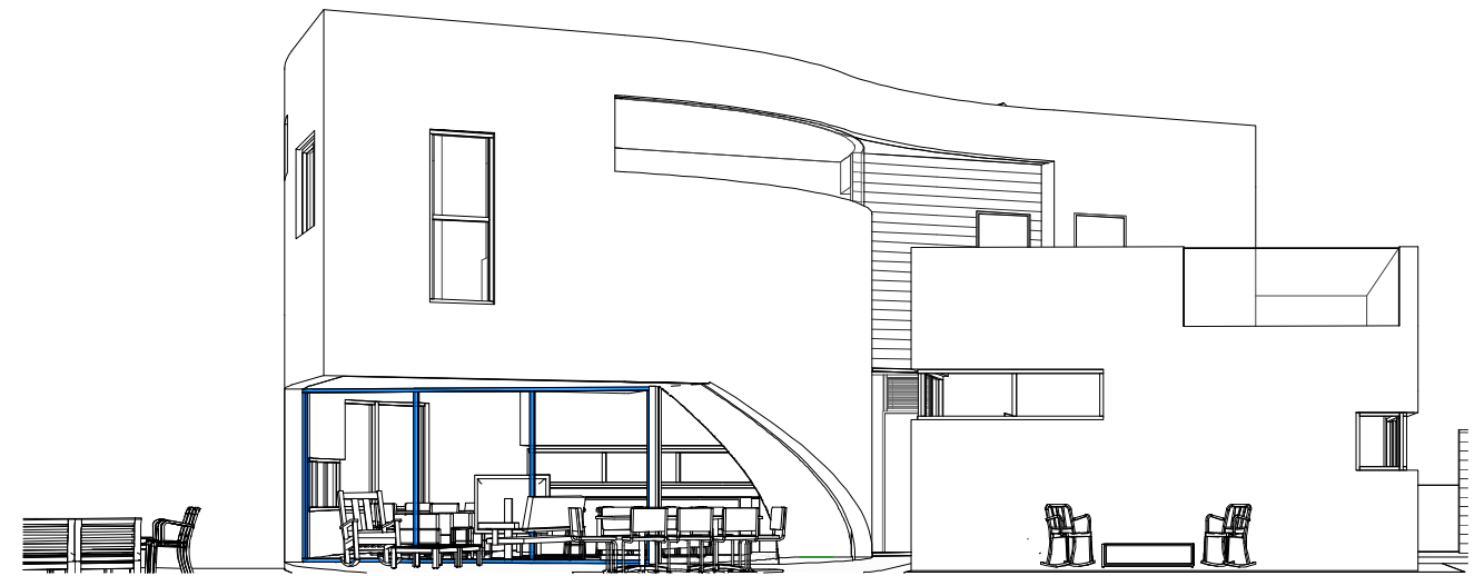
חזית דרומית
