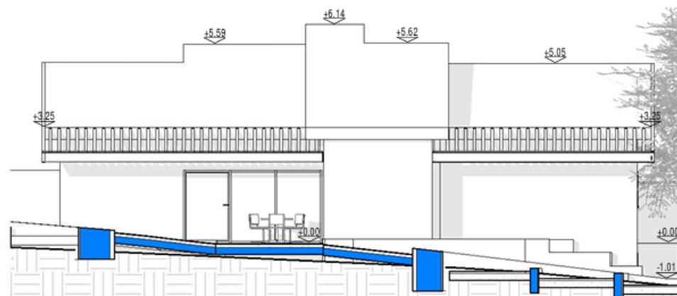
חזית מערבית
