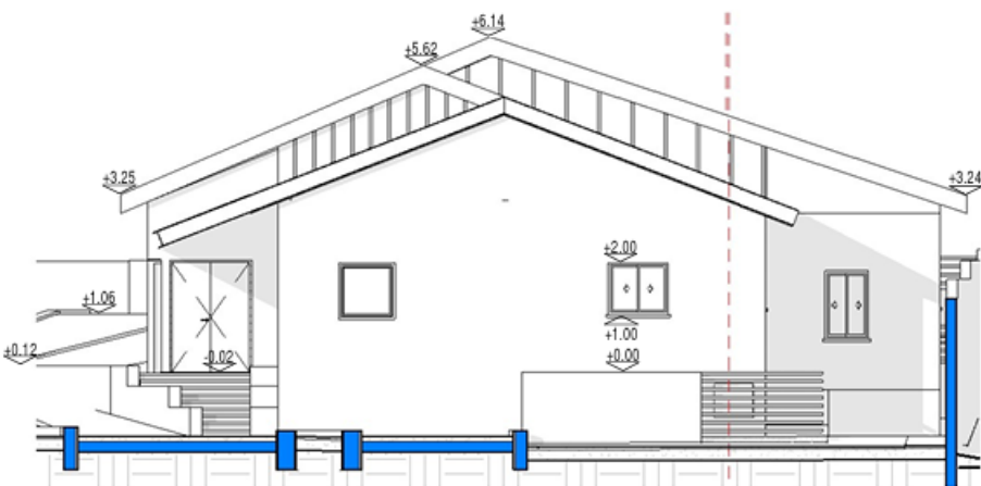
חזית מזרחית
